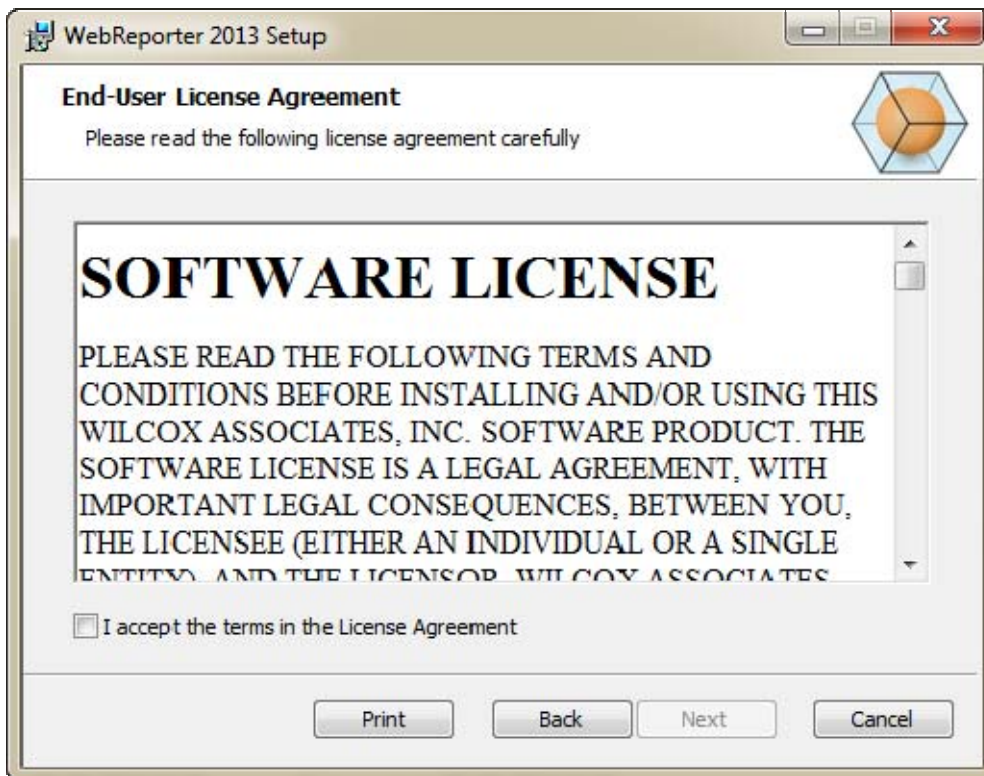
Abbildung 6 – Fenster "Endbenutzer-Lizenzvertrag"
