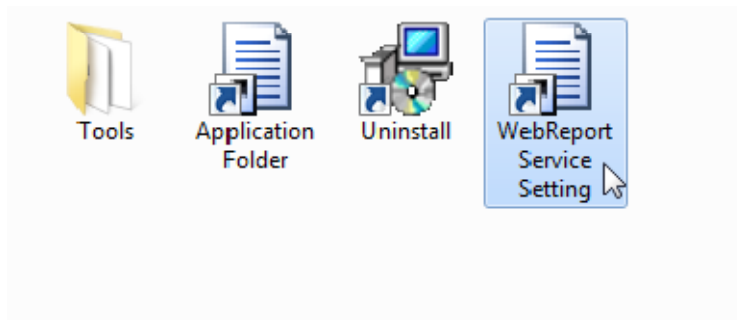
Abbildung 13 – WebReporter Programm-Verknüpfungen
