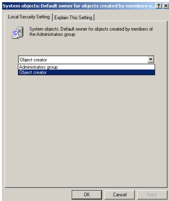
Abbildung 31 –Dialogfeld "Systemobjekte"
