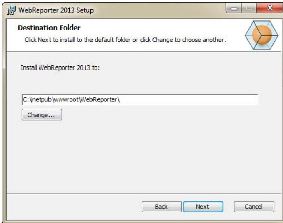
Abbildung 8 – Fenster "Zielordner"
