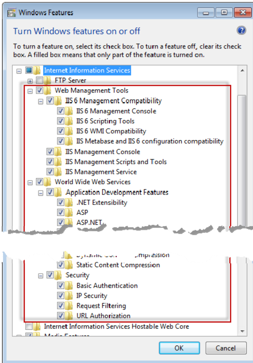
Abbildung 1 – Windows-Funktionen
