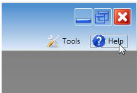
Abbildung 18 – Schaltfläche "Hilfe"
