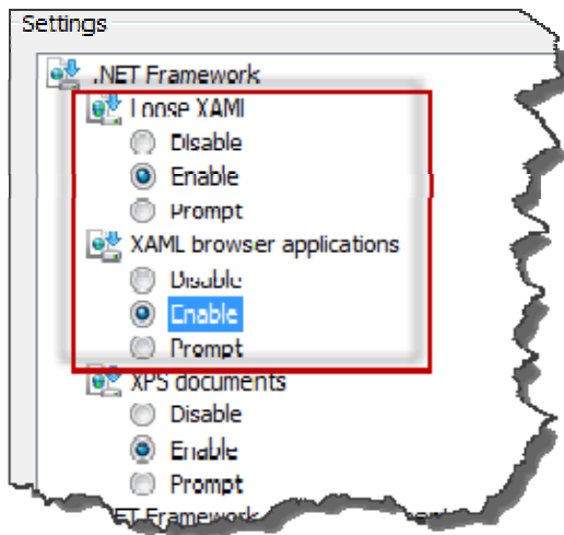
Abbildung 23 – XAML-Optionen aktivieren
