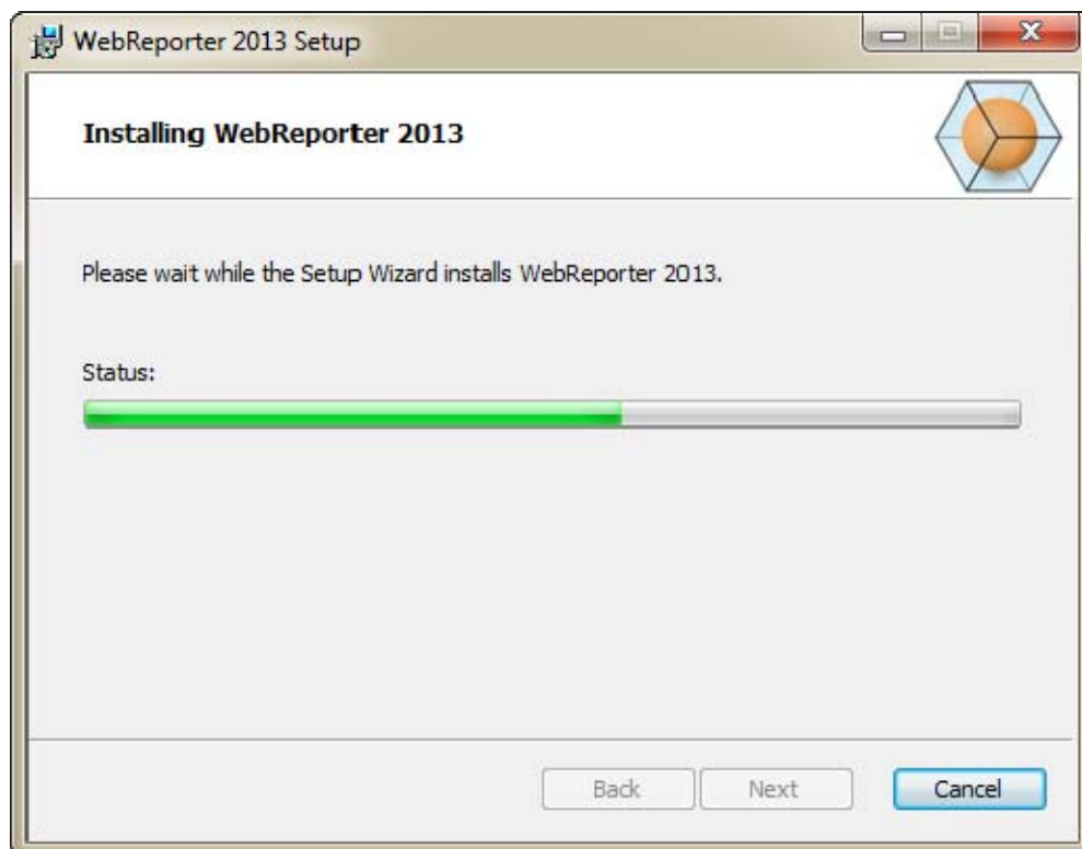
Abbildung 10 – Fenster "Installation"
